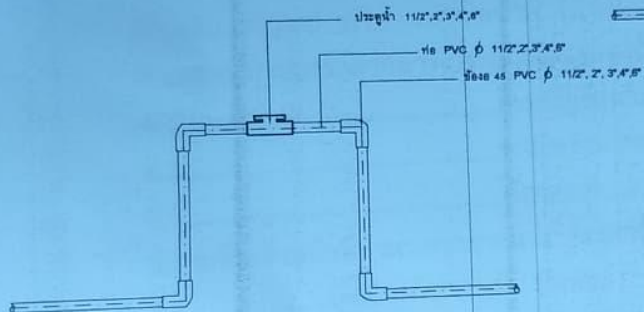
ขยายการติดตั้งประตุน้ำ
